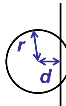
spindle torus r > d
